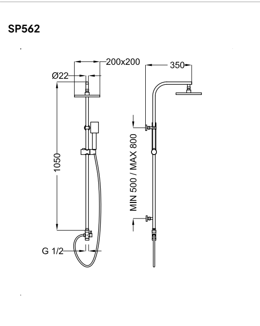
SP562 Sprchový set hranatý: bez baterie s přepínačem, sprcha 200×200 mm, sprchová růžice, hadice Shower set square without mixer with diverter, shower head 200×200mm, handshower, shower hose 2 450 CZK // 98 EUR
